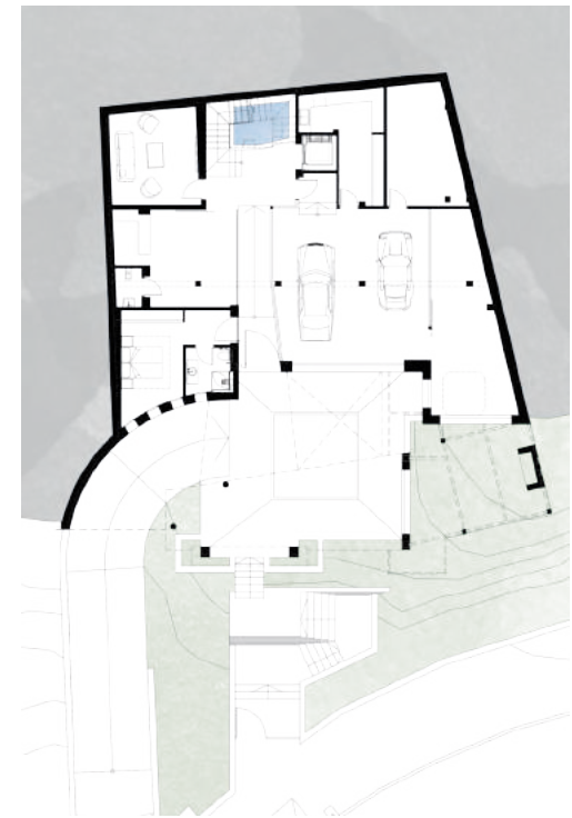
PLANTA SÓTANO BASEMENT FLOOR
